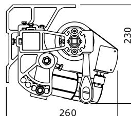
Mennyezeti rögzítés
